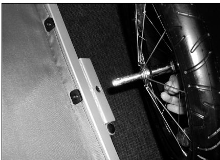
Führen Sie die Achse in die Aufnahme am Vierkantrahmen ein.
