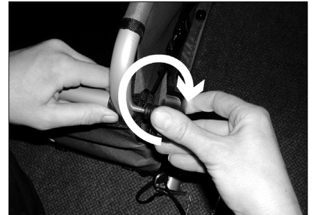
Beide Querrohre mit den an Bändchen befestigten Sterngriffbolzen festschrauben.
