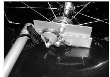
Verriegeln Sie den Bolzen durch Umlegen des Federclips. Der Bügel muss nach dem Schliessen den Bolzen umschliessen.
